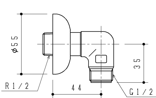
リモデル壁給水用エルボ
