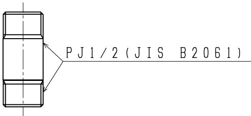
リモデル床給水用ニップル
