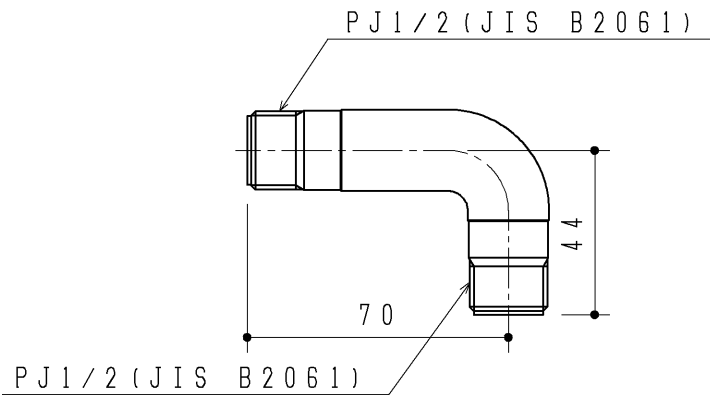
リモデル壁給水用エルボ
